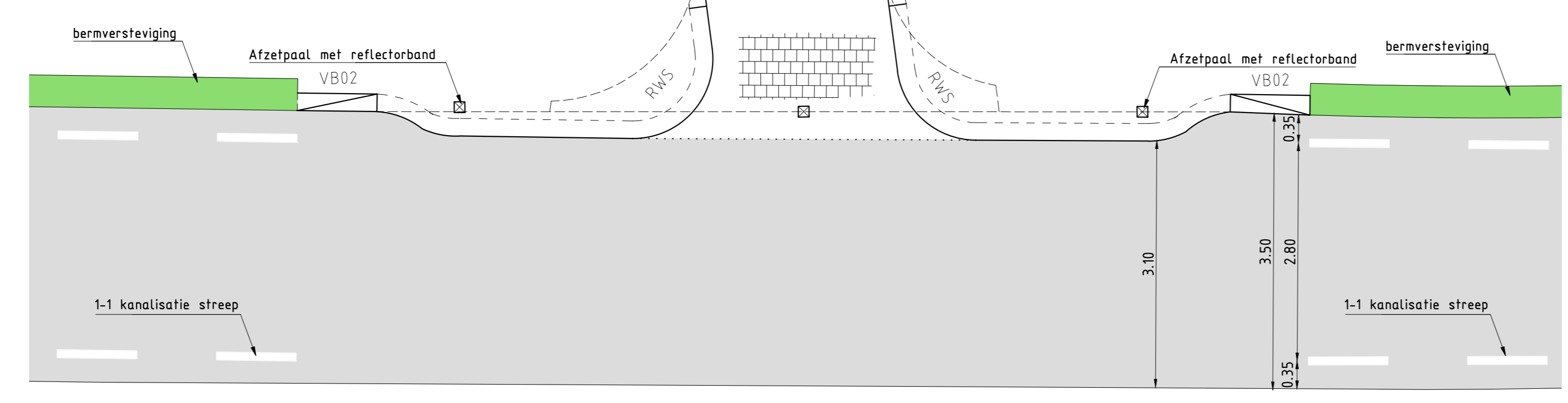
Aanluiting fietspaden SCHAAL 1:50
